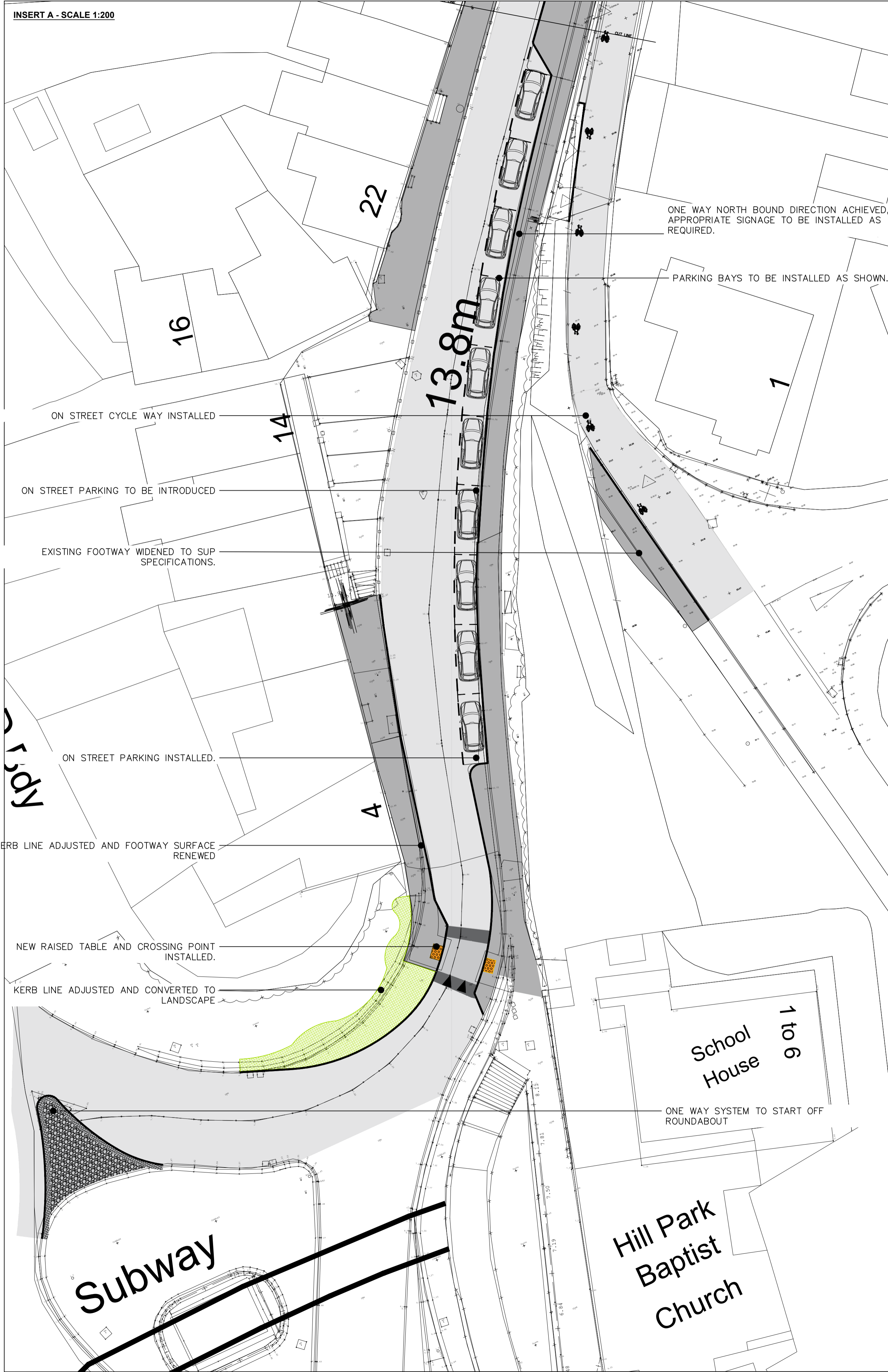
INSERT B - SCALE 1:200
